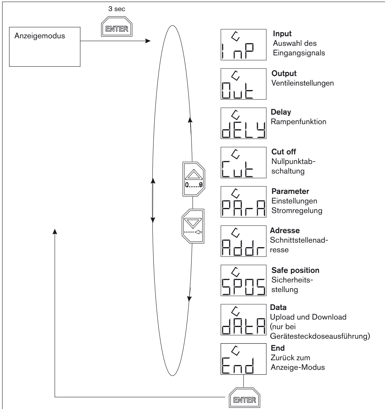
Bild 14: Menü des Konfigurationsmodus
