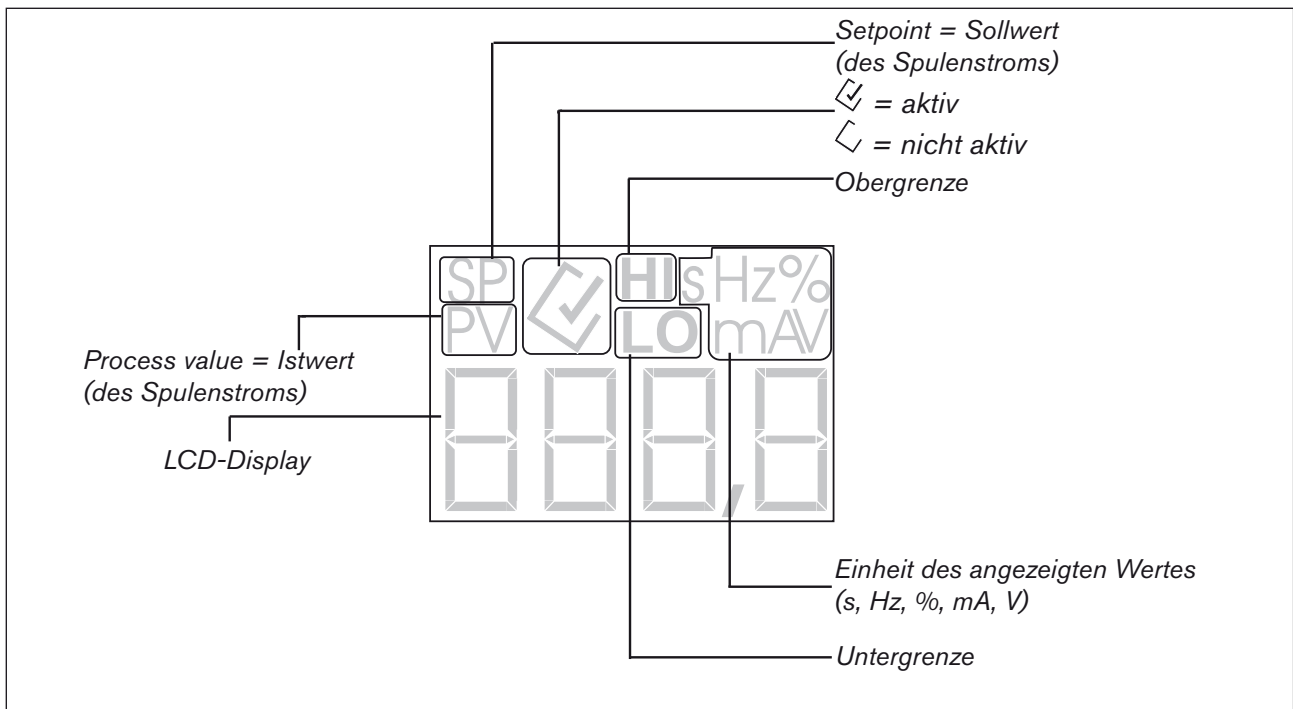
Bild 3: Bedieneinheit
