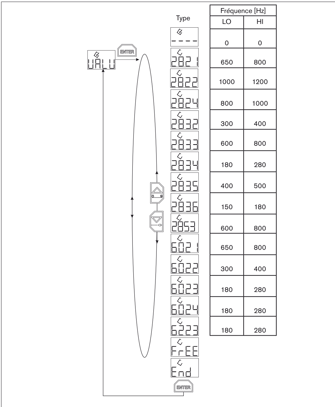
Figure 18 : Fréquences limites pour les types de vannes Bürkert
