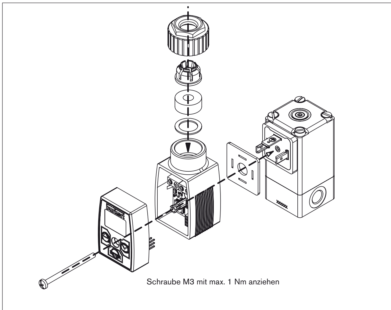
Bild 11: Montage der Gerätesteckdoseausführung an das Ventil
