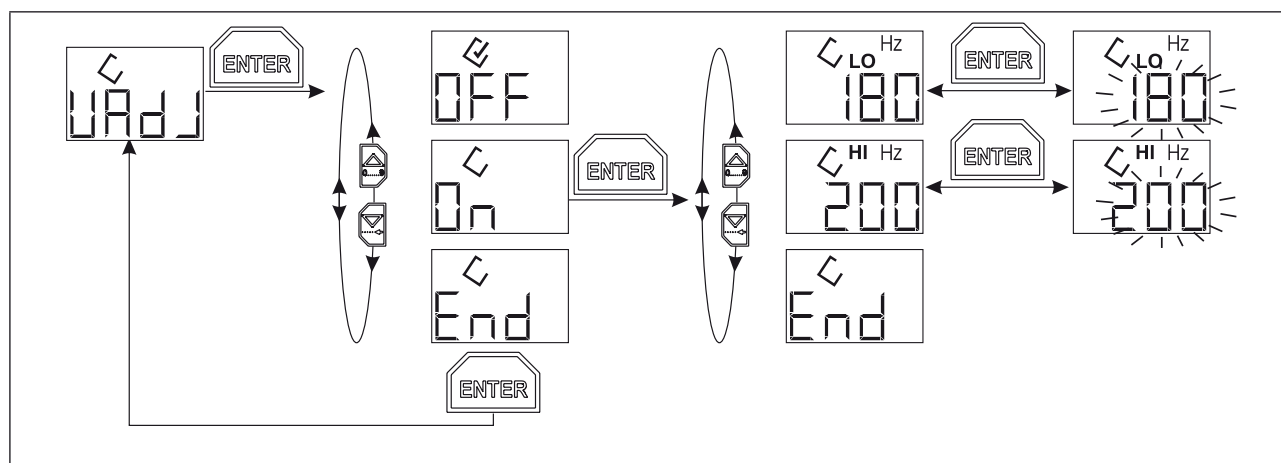
Figure 19 : VAdJ (Valve adjust) - Syntonisation précise de la fréquence de vanne
