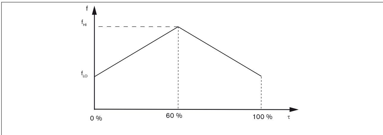
Bild 17: PWM-Frequenz / Tastverhältnis
