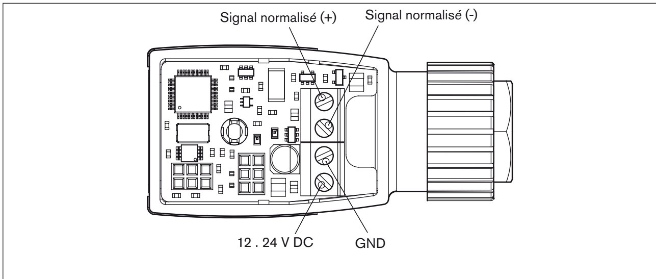
Figure 9 : Raccordement sur la borne plate
