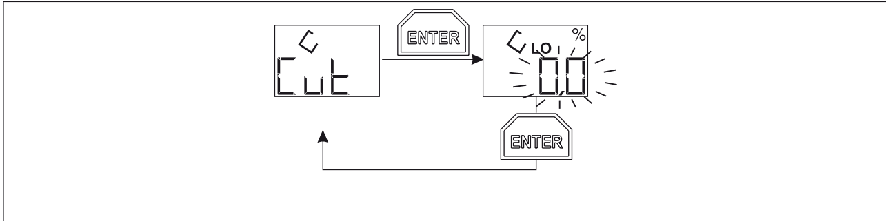
Bild 22: Cut (Cut off) - Nullpunktabschaltung
