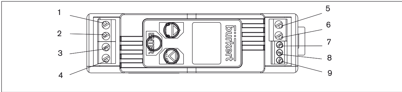
Bild 12: Anschluss Klemmleiste
