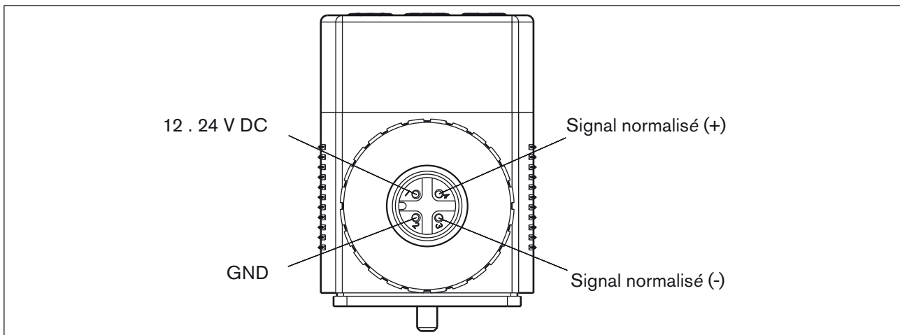
Figure 10 : Raccordement sur le connecteur
