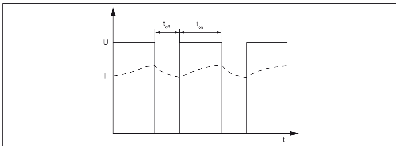
Bild 6: Zeitverlauf von PWM-Spannungssignal aus Spulenstrom
