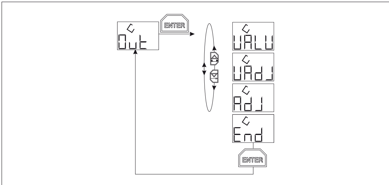
Figure 16 : Out (Output) - Réglages de la vanne
