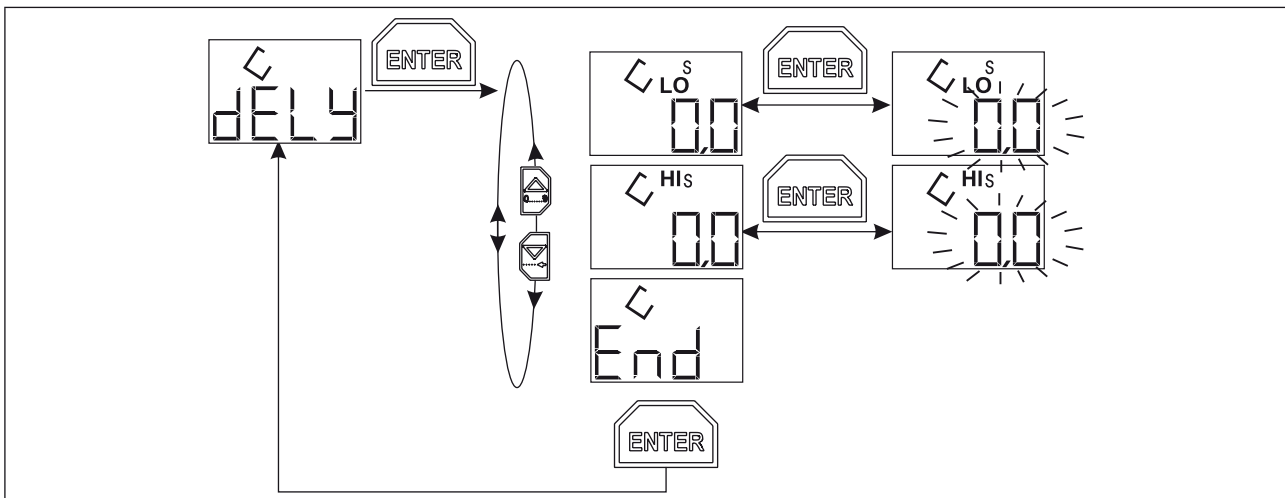
Figure 21 : dELY (Delay) - Fonction de rampe
