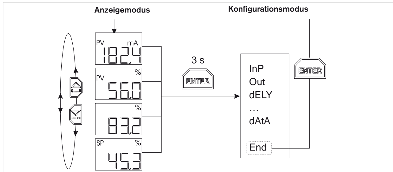
Bild 13: Wechsel zwischen Anzeige- und Konfigurationsmodus
