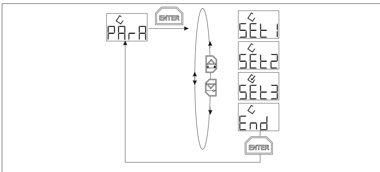
Bild 23: PArA (Parameter) - Reglereinstellung
