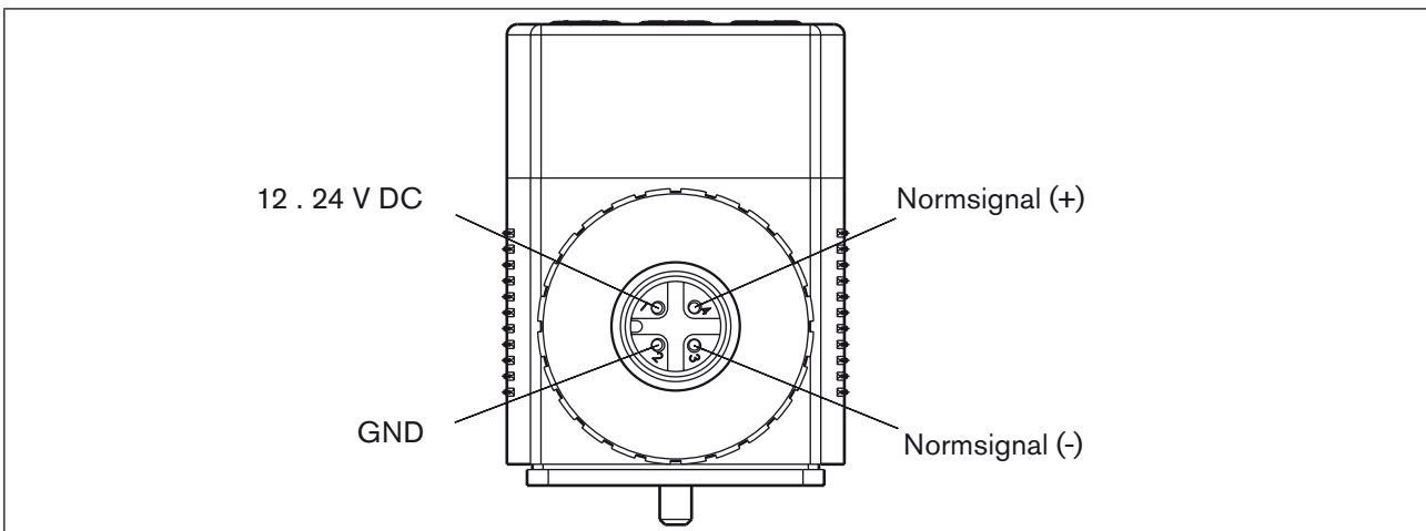
Bild 10: Anschluss Steckverbinder
