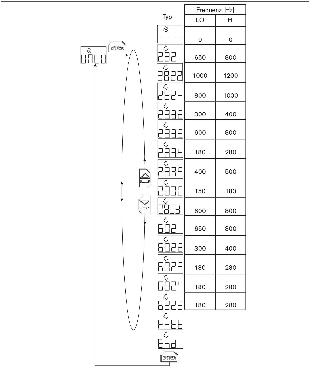
Bild 18: Grenzfrequenzen für Bürkert-Ventiltypen
