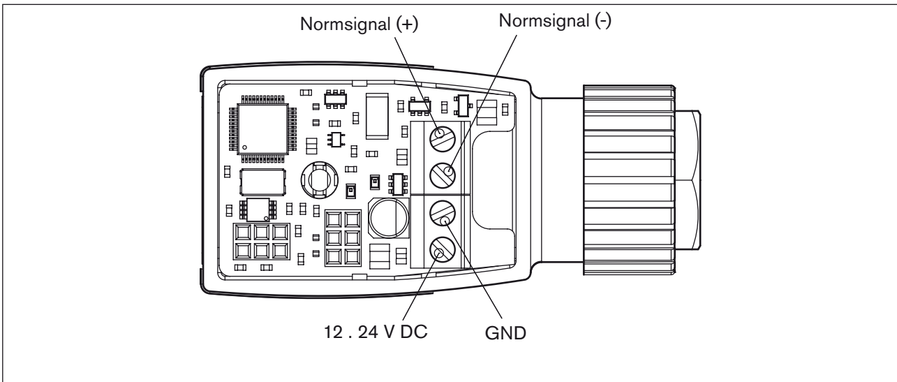
Bild 9: Anschluss Klemmleiste
