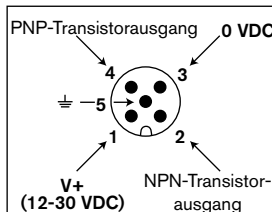
NPN/PNP-Anschluss des M12-Gerätesteckers
