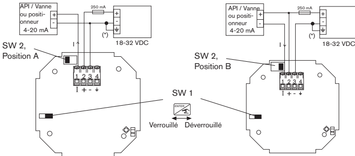
Fig. 3.15 Affectation des broches, Position A Fig. 3.16 Affectation des broches, Position B
