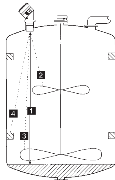
Fig. 4.1 Filtrage des échos
