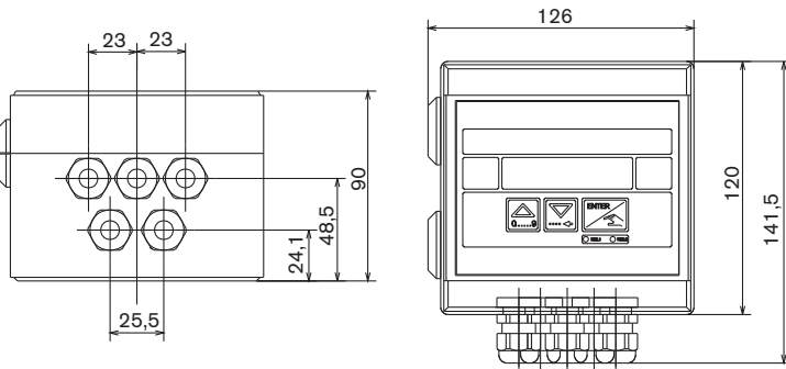
Version murale (en mm)
