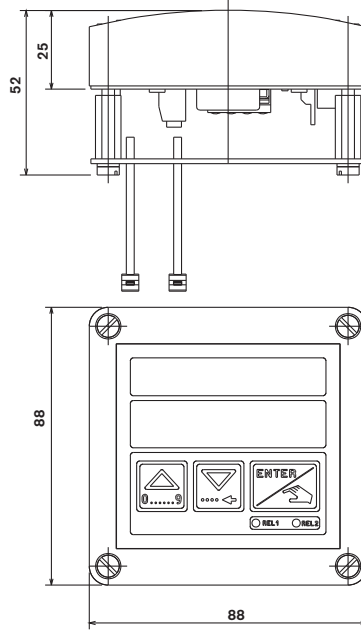
Version encastrable (en mm)
