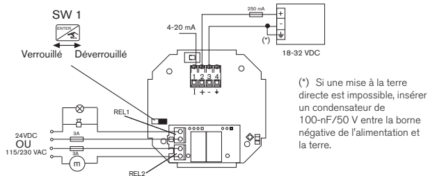
Fig. 3.7 Affectation des bornes des relais
