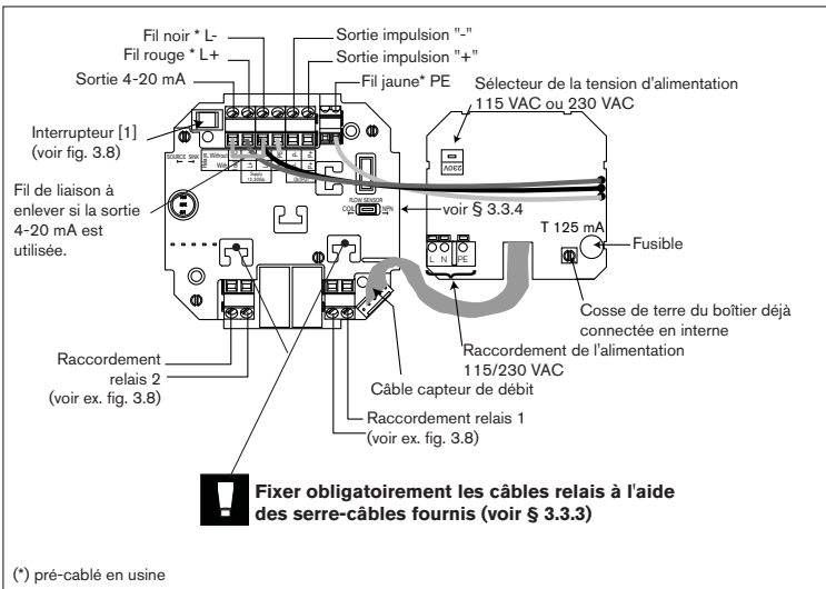
Fig. 3.12 Connexion SE35, 115/230 VAC, avec relais et presse-étoupes
