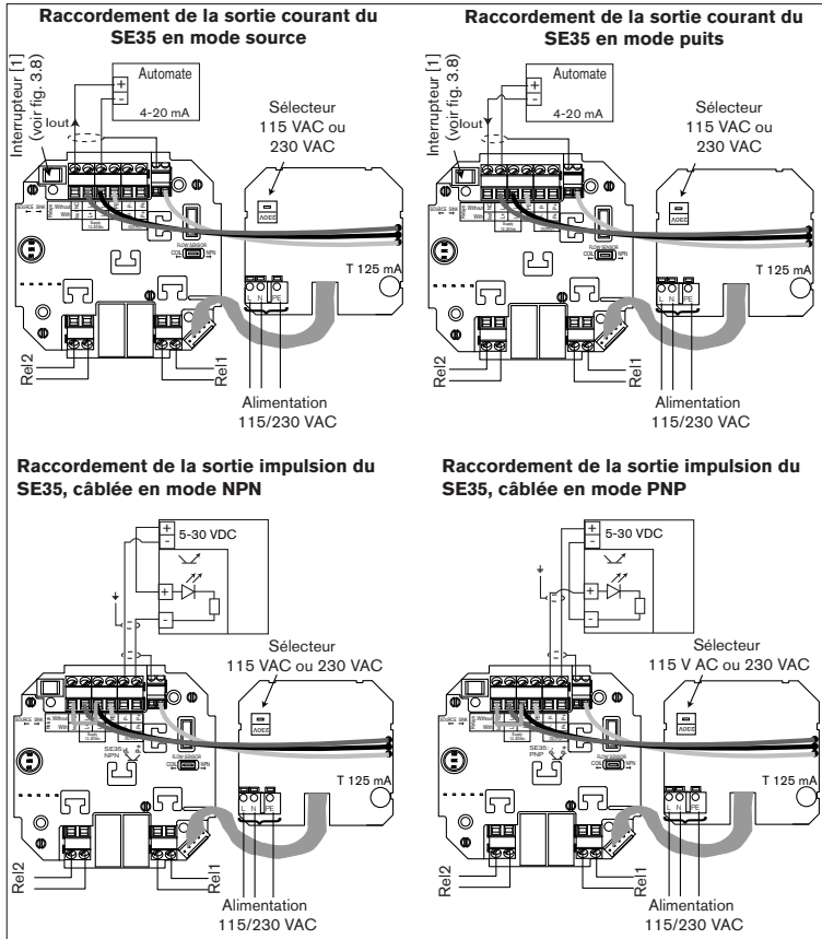
Fig. 3.13 Raccordement du module électronique SE35, 115/230 VAC, avec relais et presse-étoupe, à un automate
