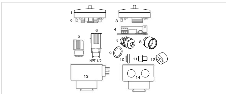
Fig. 5.1 Ersatzteil-Explosionszeichnung SE35
