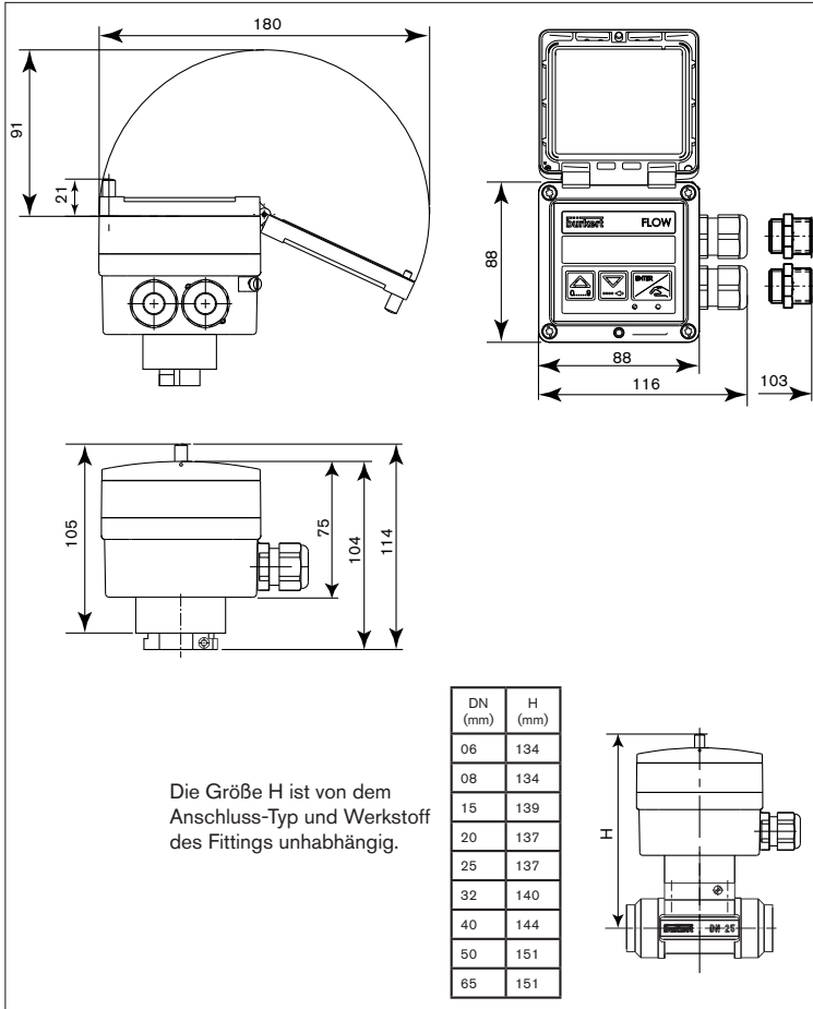
Fig. 2.1 Durchfluss-Transmitter Abmessungen
