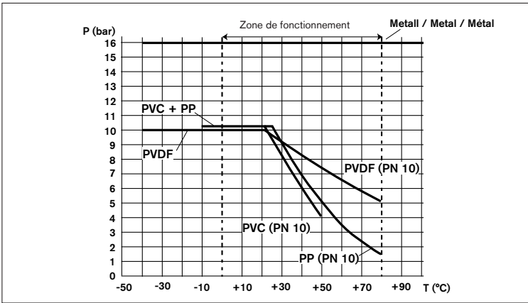
Fig. 3.1 Dépendance température-pression
