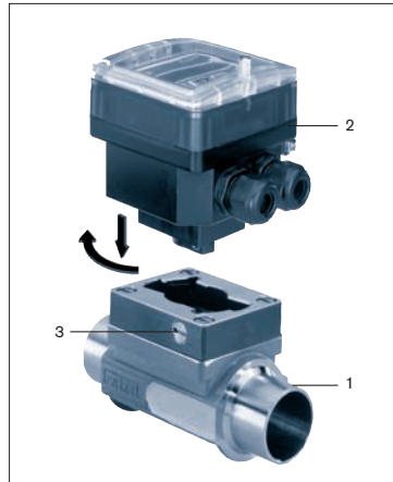
Fig. 3.2 Einbau 8035
