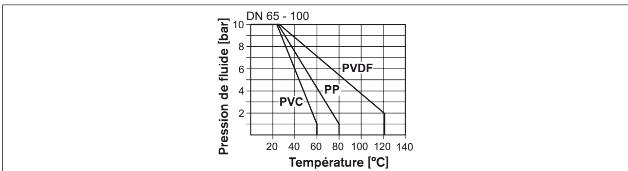
Figure 2 : Diagramme pression de fluide / température de fluide
