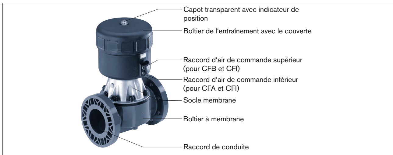
Figure 7 : Structure et description
