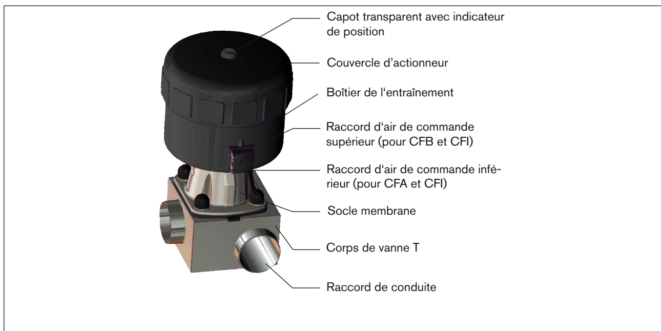
Figure 8 : Structure et description Type 2032
