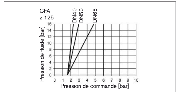
Fig. 17 : Diagramme de pression, actionneur ø 125, fonction de commande A
