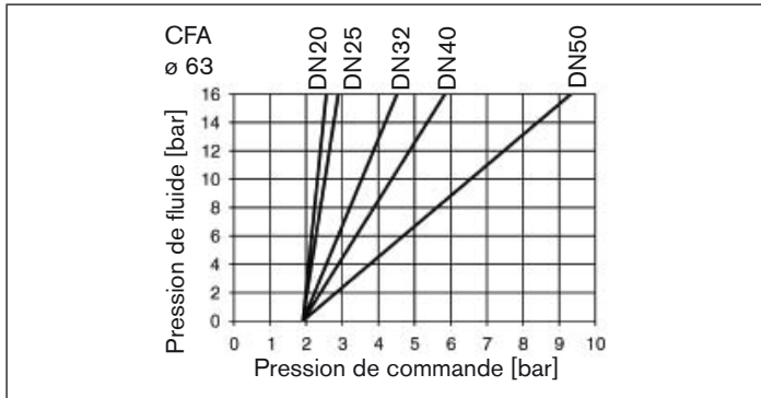
Fig. 14 : Diagramme de pression, actionneur ø 63, fonction de commande A
