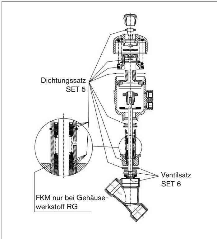
Bild 22: Ersatzteile Schrägsitzventil
