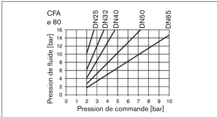
Fig. 15 : Diagramme de pression, actionneur ø 80, fonction de commande A
