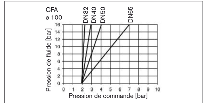
Fig. 16 : Diagramme de pression, actionneur ø 100, fonction de commande A
